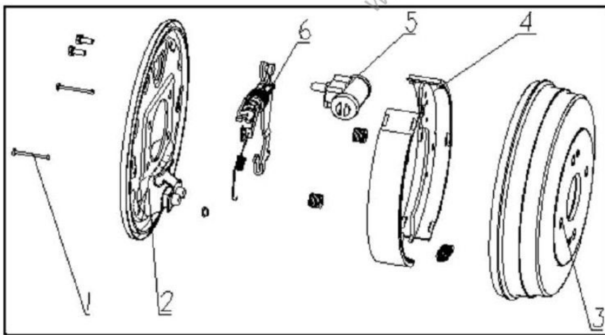
(1) 前弹簧座杆 (2) 后制动底板 (3) 制动鼓 (4) 后制动蹄 (5) 后制动分泵总成
